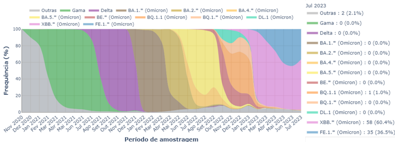
Figura 3. Linhagens relevantes do SARS-CoV-2 ao longo do tempo. Brasil, novembro de 2020 a julho de 2023.
