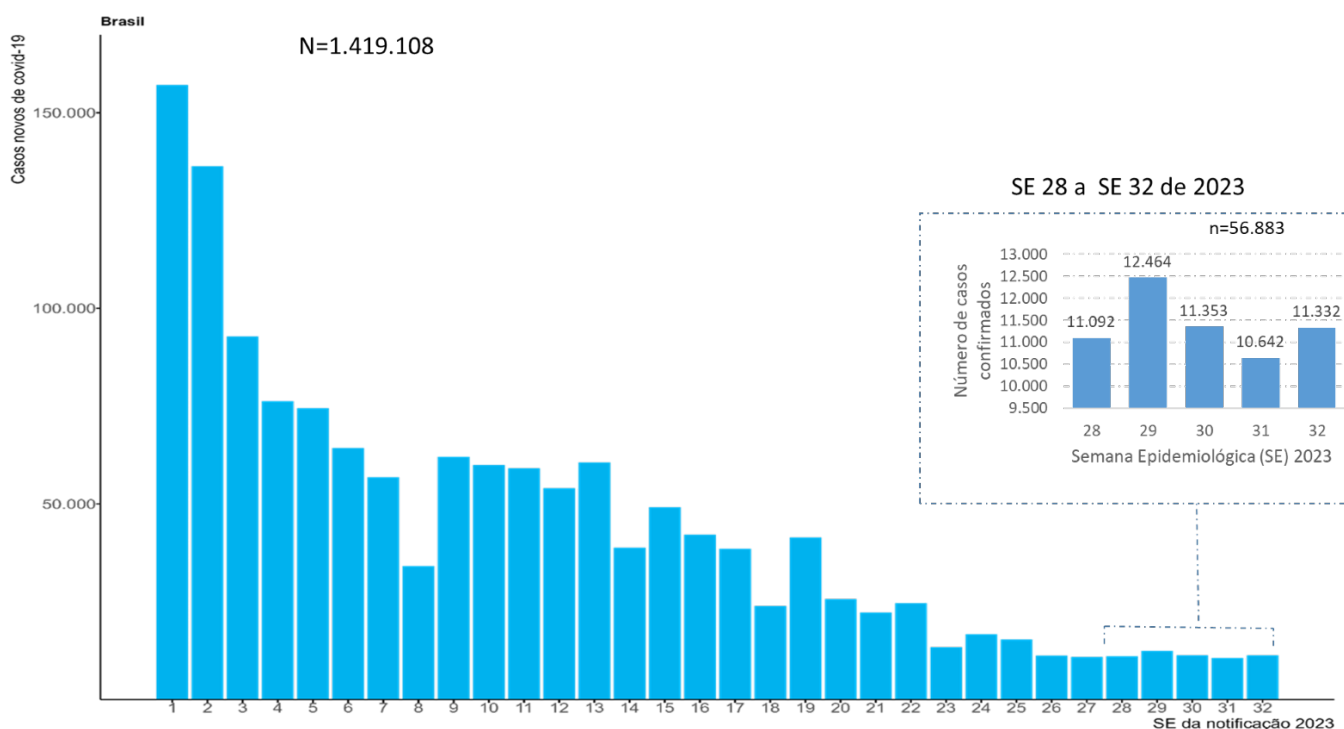
Figura 1 - Distribuição dos casos por covid-19, segundo Semana Epidemiológica por data de notificação, Brasil, 2023
