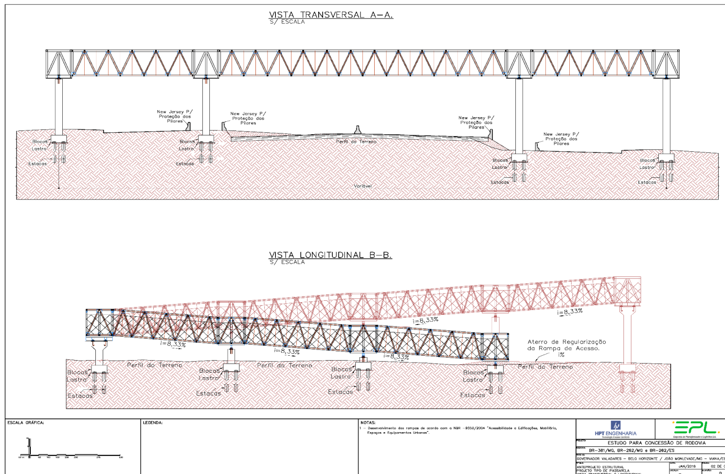
Figura 36 – Croqui Básico Passarela
