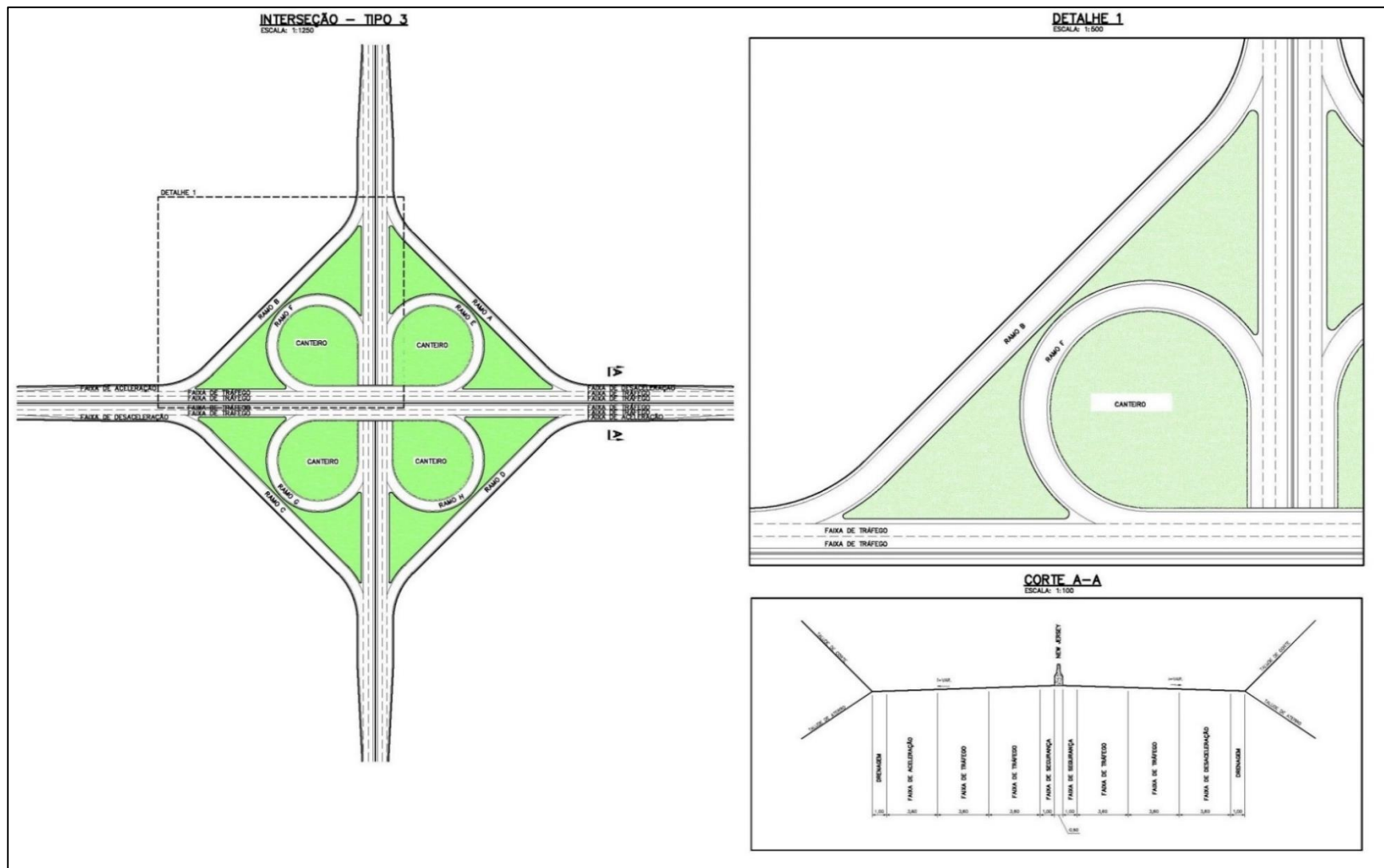
Figura 46 – Croqui Básico Trevo
