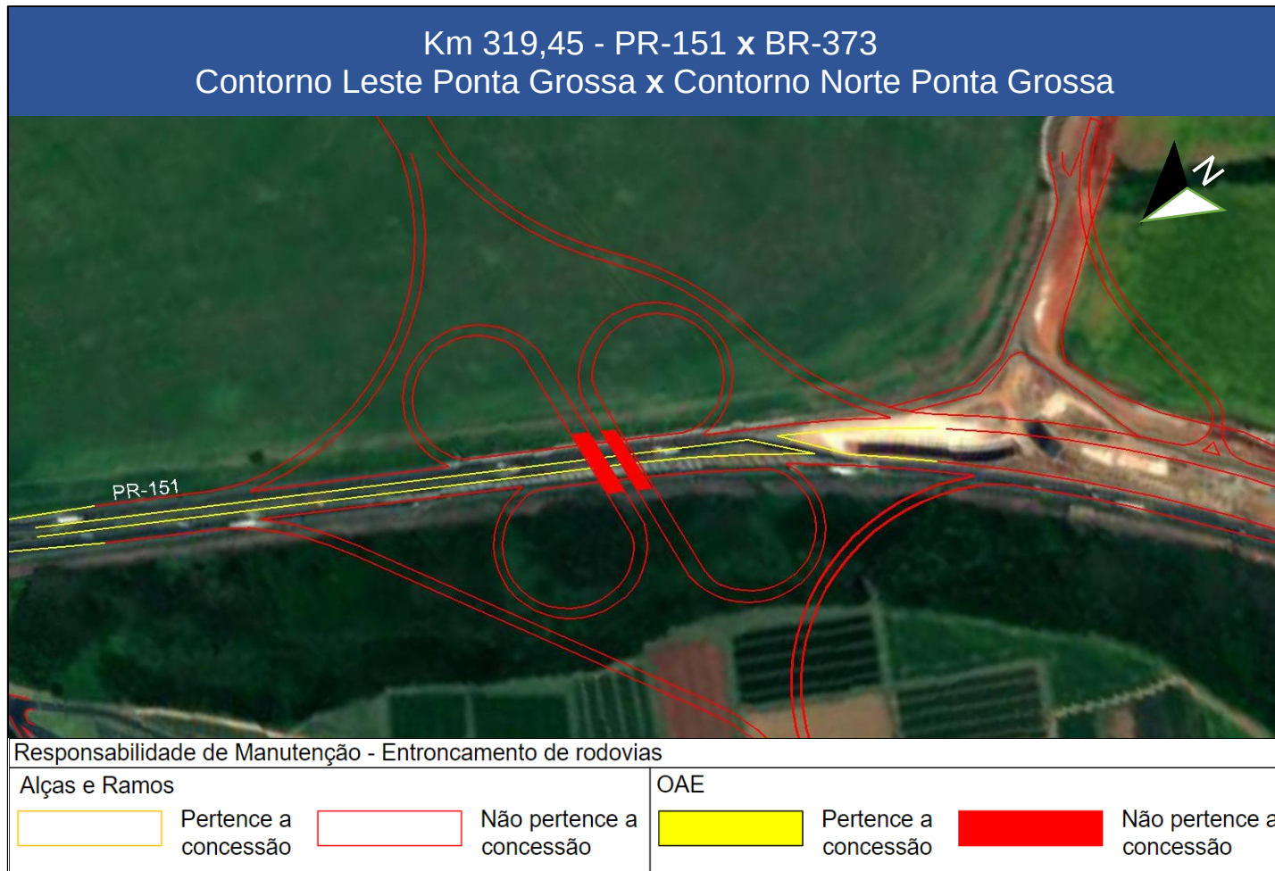
Figura 78 – Interseções PR-151 x BR-373 – km 319,45
