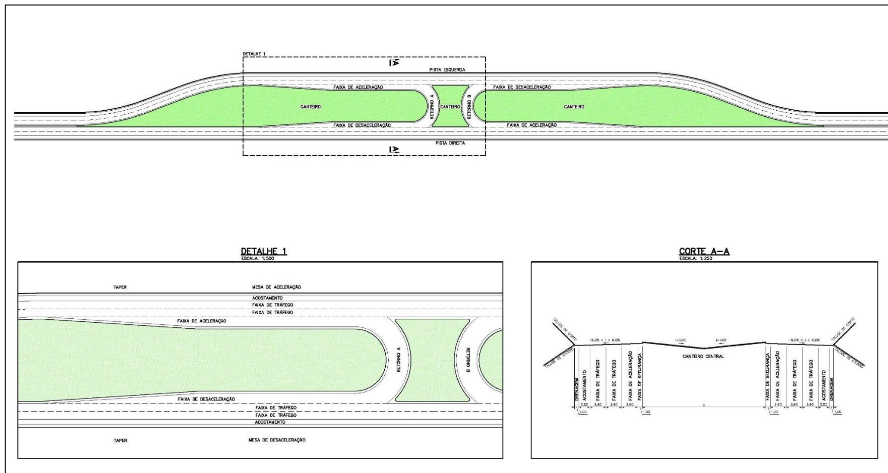
Figura 40 – Croqui Básico Retorno em X
