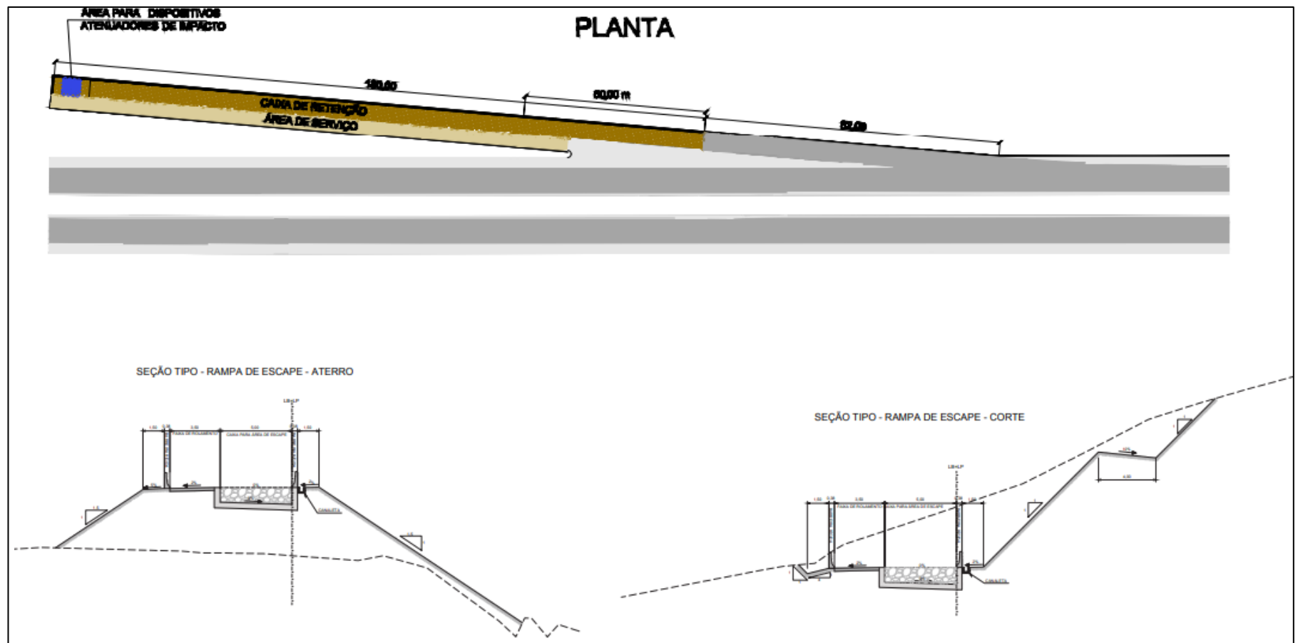
Figura 48 – Croqui Básico Área de Escape
