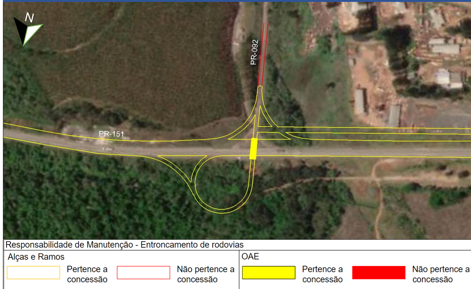
Figura 72 – Interseções PR-151 – Entroncamento com PR-092
