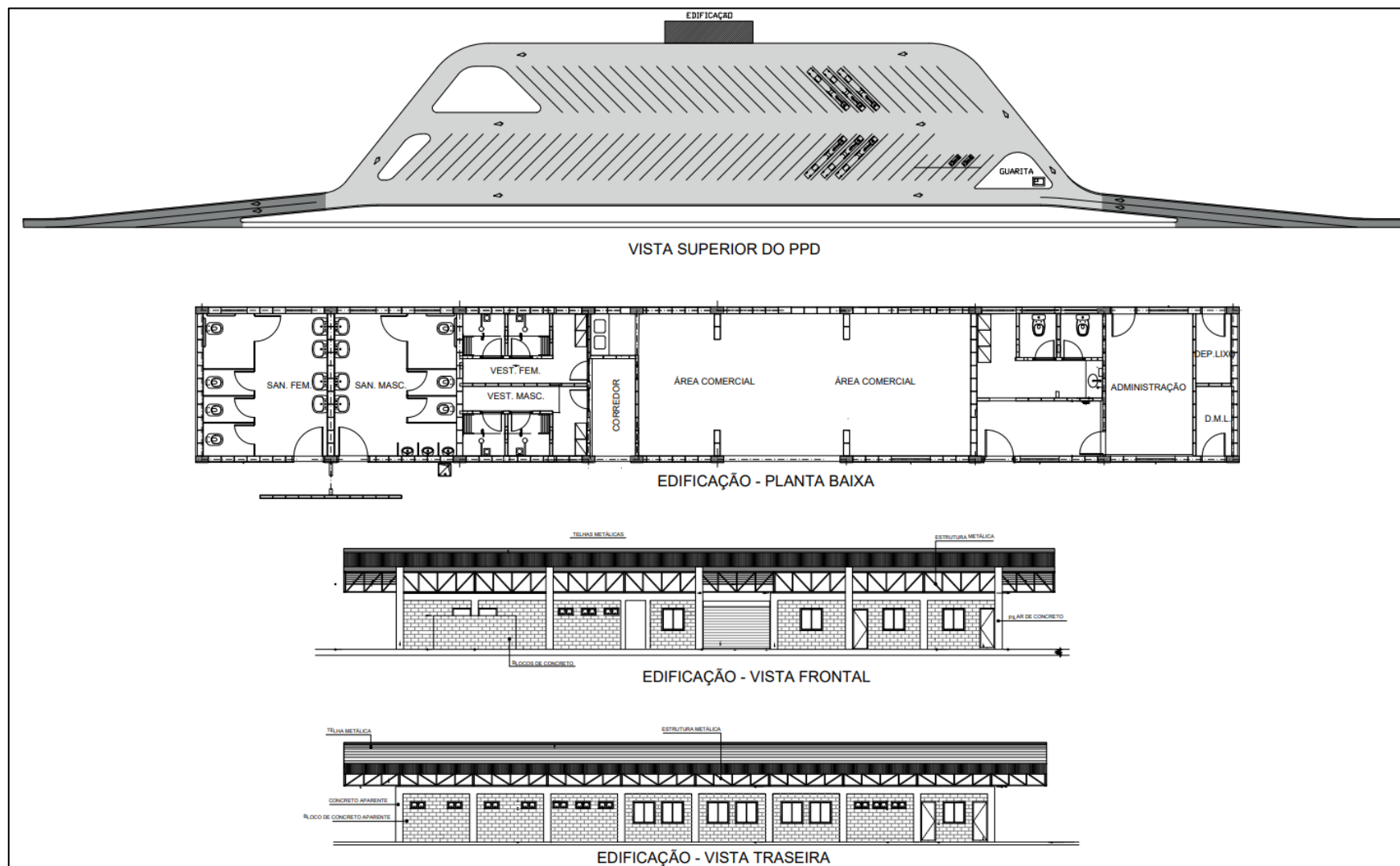
Figura 47 – Croqui Básico Ponto de Parada e Descanso (PPD)
