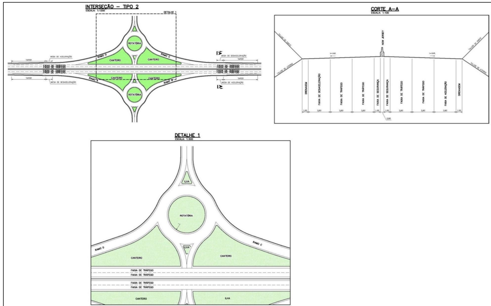
Figura 45 – Croqui Básico Diamante
