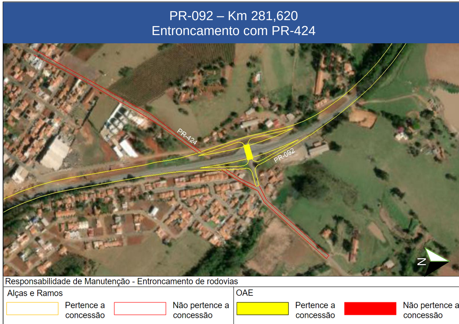
Figura 66 – Interseções PR-092 – Entroncamento com PR-424
