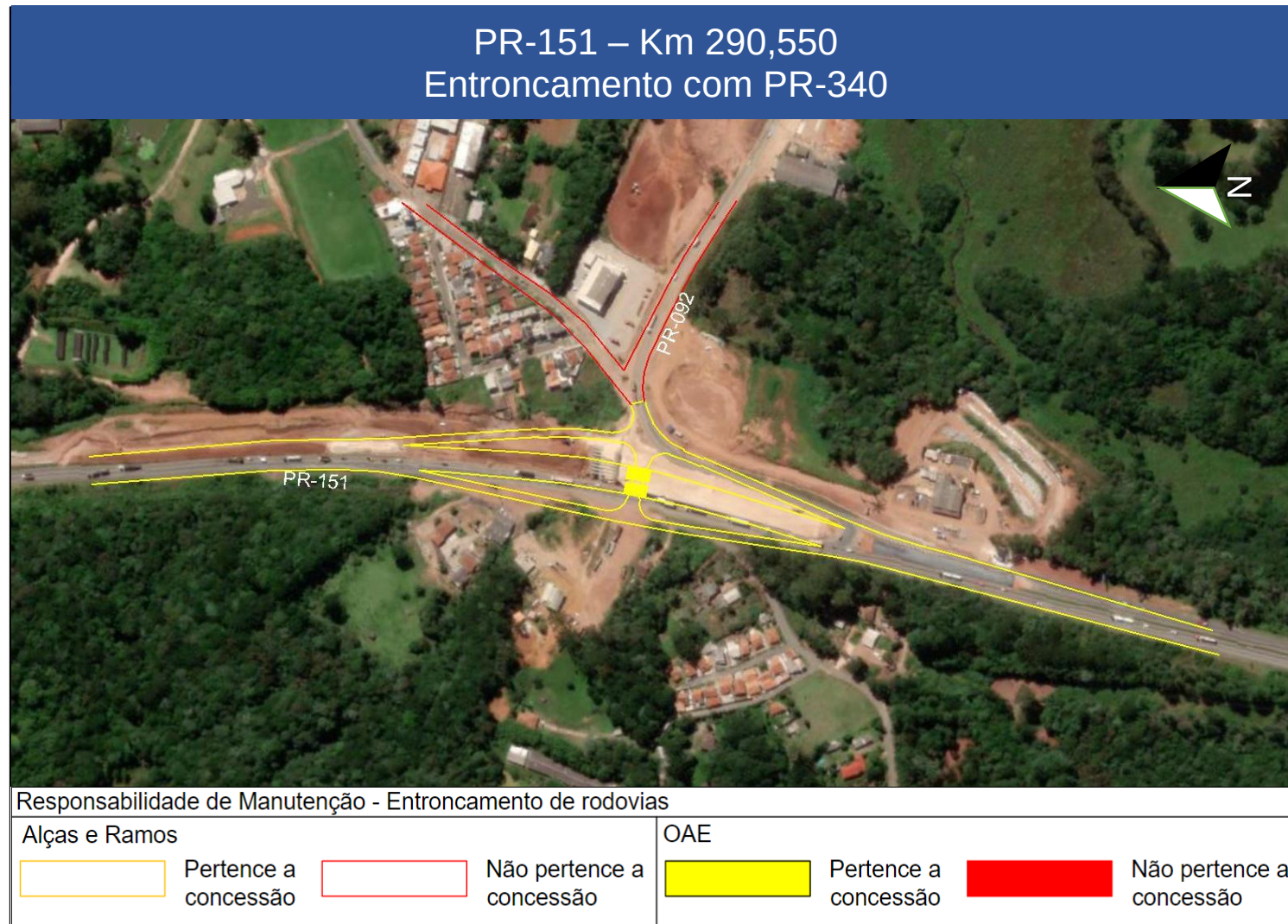
Figura 76 – Interseções PR-151 – Entroncamento com PR-340
