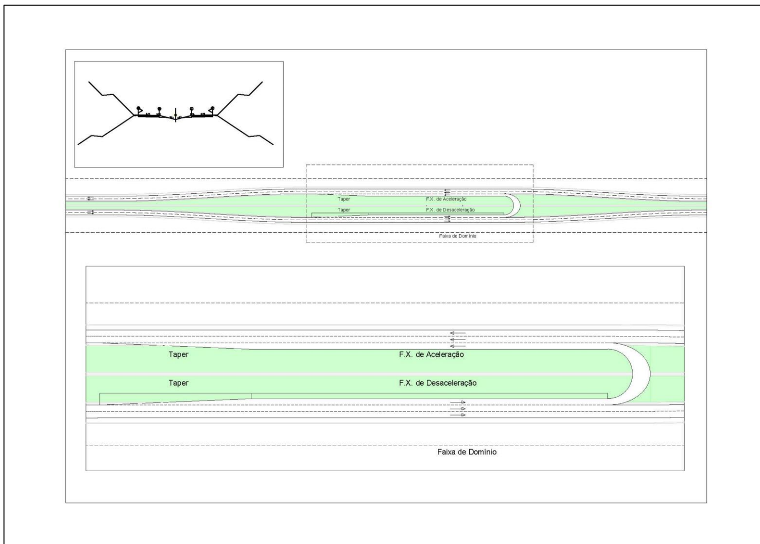
Figura 41 – Croqui Básico Retorno em U
