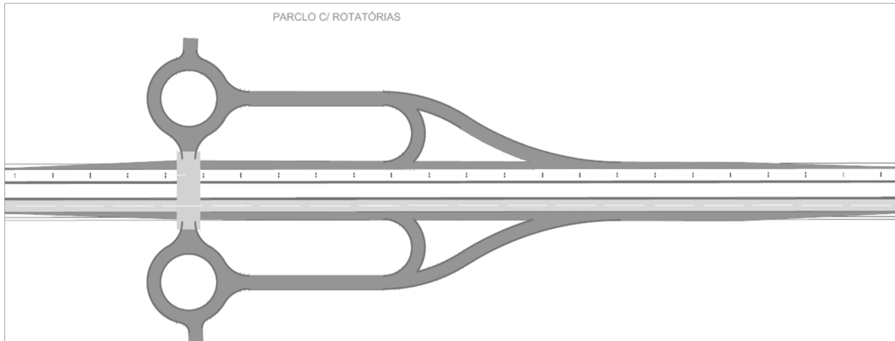
Figura 43 – Croqui Básico Parclo com Rotatória
