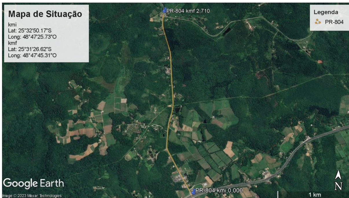
Figura 33 – Segmento da PR-804: Início no Entr. com PR-277/PR km 0,00 e Final no Entr. com a PR-408 km 2,710
