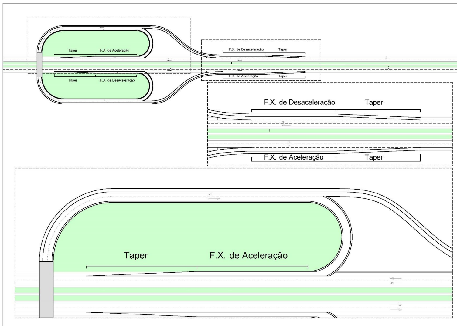
Figura 42 – Croqui Básico Parclo sem Rotatória
