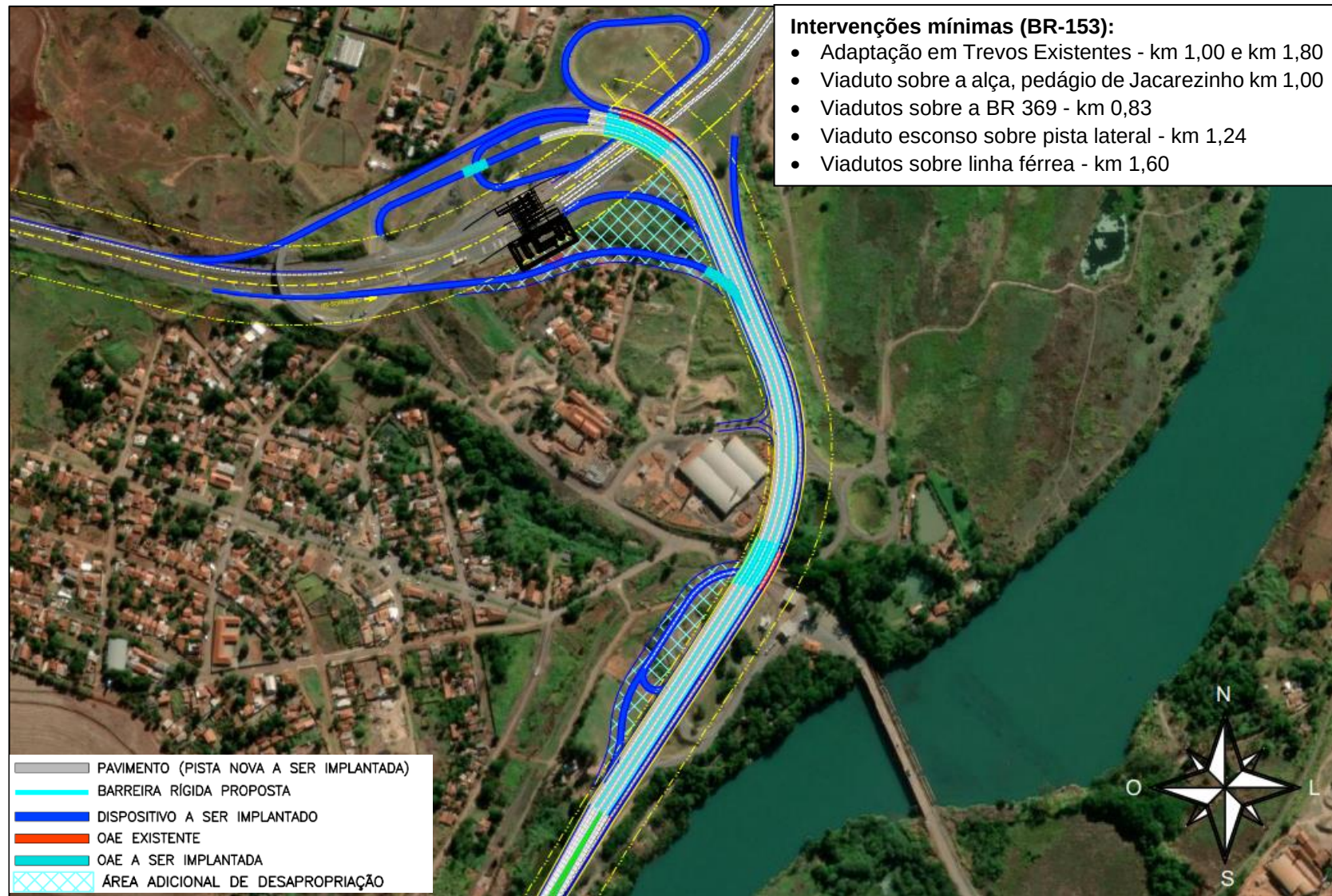
Figura 89 - Intervenções mínimas no entorno da Praça de Pedágio Jacarezinho I - km 1,000 da BR 153/PR
