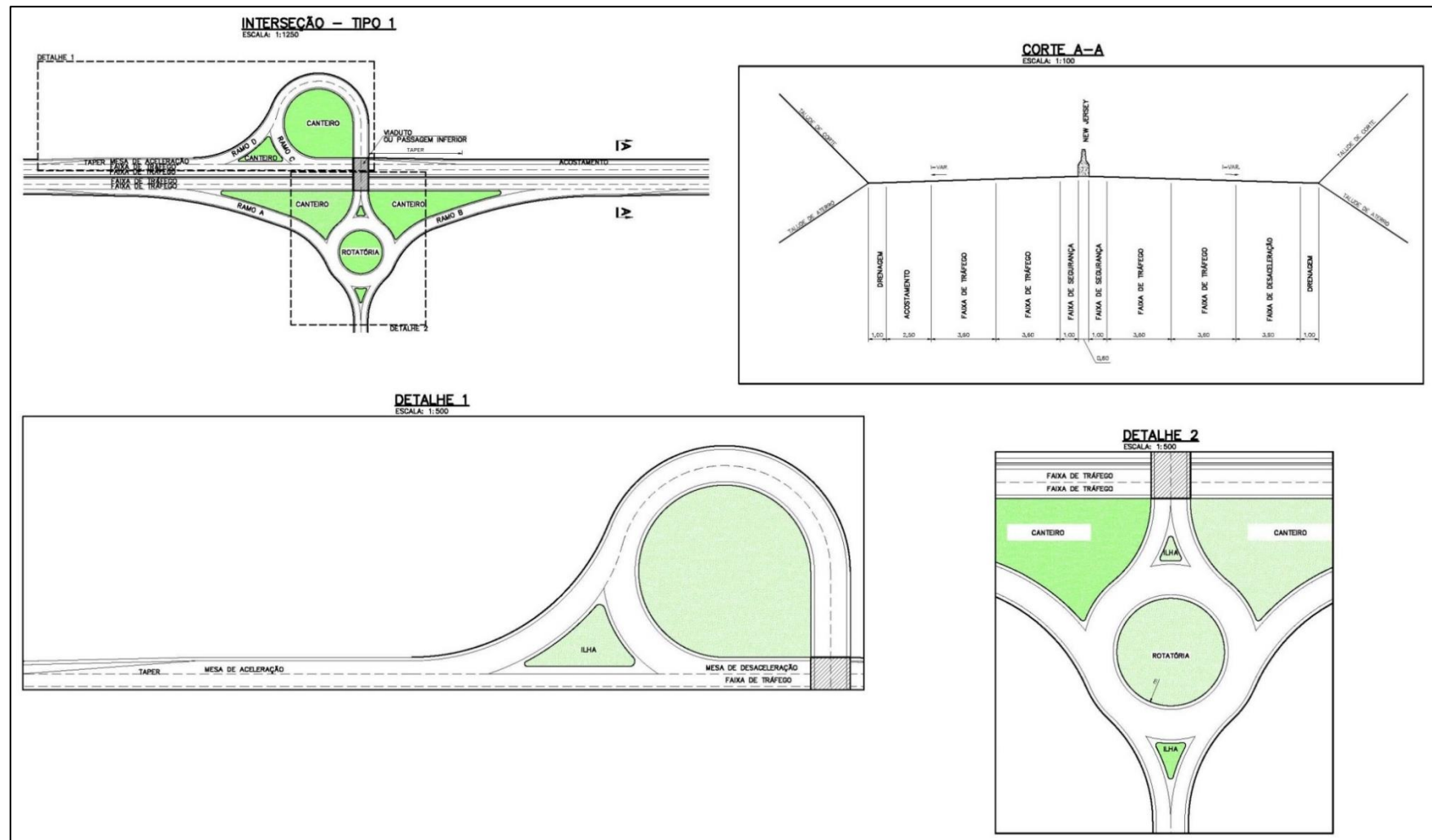
Figura 44 – Croqui Básico Trombeta
