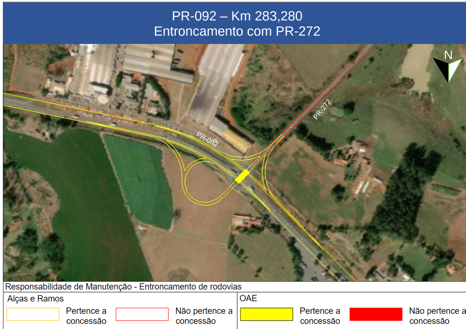
Figura 67 – Interseções PR-092 – Entroncamento com PR-272
