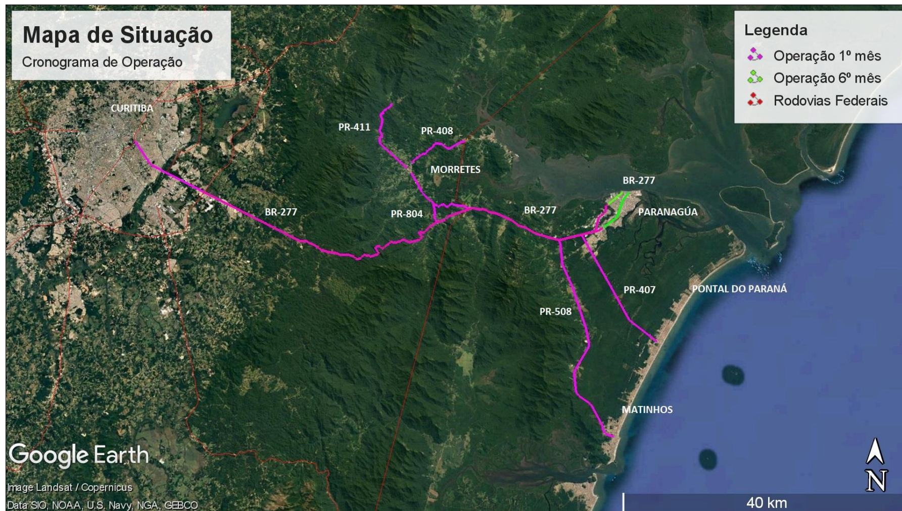
Figura 4 – Mapa de Implantação Operacional – Malha Sul
