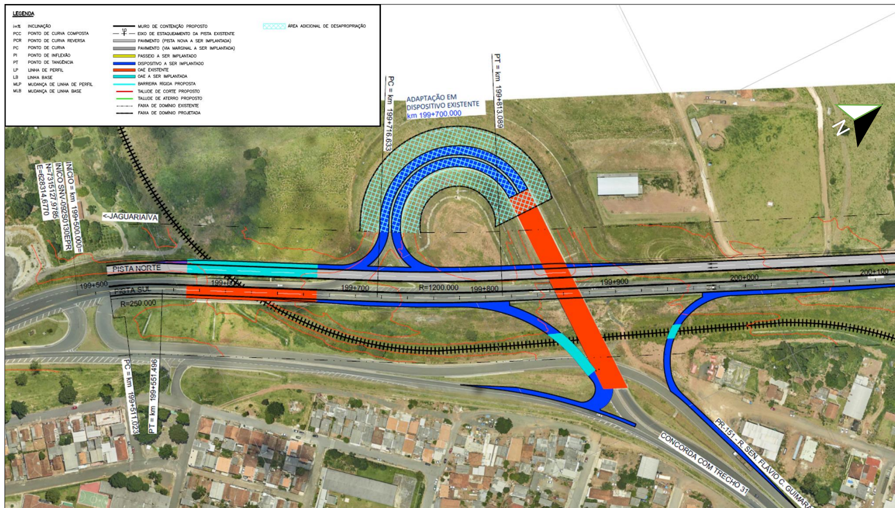
Figura 88 – Dispositivo Especial – Rede Ferroviária Federal – PR-092
